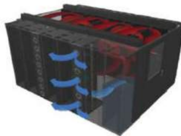
Sistema de contención térmica ENCLOSURE
